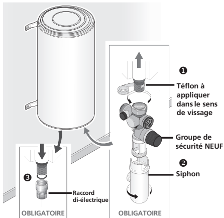
Branchement eau chaude Branchement eau froide
